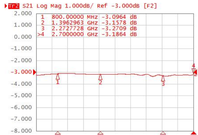
图2 插入损耗
