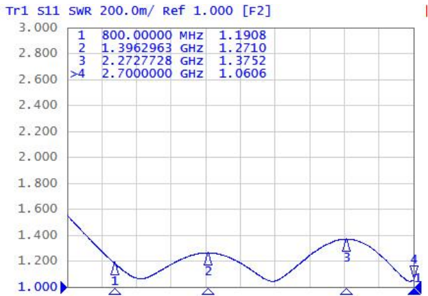
图1 合路端驻波比
