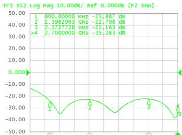
图3 隔离度
